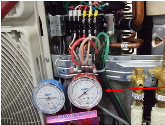
ガス圧測定
