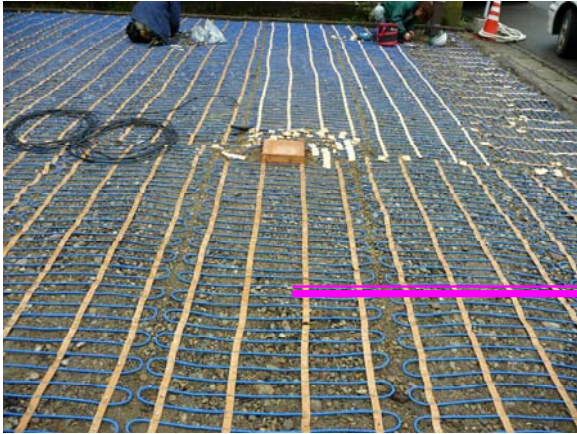
電熱線敷設
