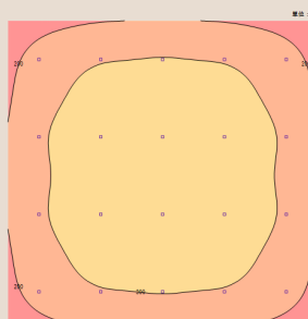
照度分布図(LED)
