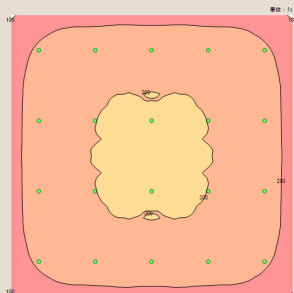
照度分布図(水銀灯)
